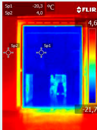
Thermografisch warmtebeeld
